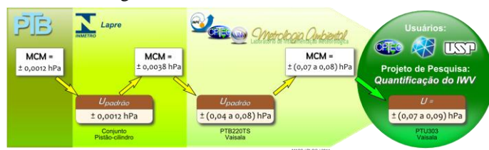
Fig. 3. A disseminação da variável pressão atmosférica
