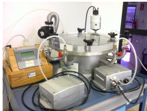
Fig. 6. Sistemas de calibração de pressão atmosférica do INPE/CPTEC/LIM
