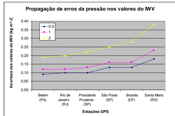
Fig. 5. Incertezas de pressão atmosférica versus incertezas nos valores de IWV
